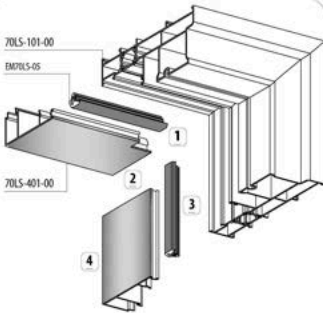
E NOCH / KERTME A B CORNER DETAIL / KÖŞE DETAYI
