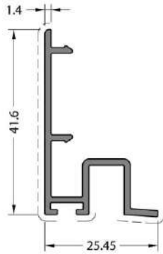
CODE / KOD 23-501-014 THEORETICAL WEIGHT kg/m TEORİK AĞIRLIK kg/m 0.366
