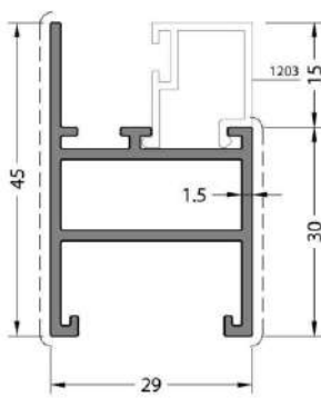
CODE / KOD 23-201-015 THEORETICAL WEIGHT kg/m TEORİK AĞIRLIK kg/m 0.579
