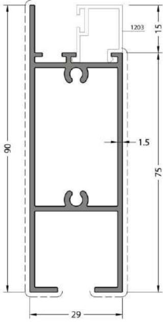
CODE / KOD 23-202-015 THEORETICAL WEIGHT kg/m TEORİK AĞIRLIK kg/m 1.068
