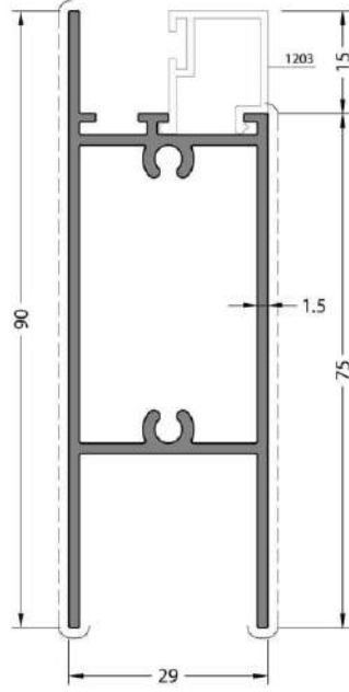
CODE / KOD 23-203-015 THEORETICAL WEIGHT kg/m TEORİK AĞIRLIK kg/m 1.010
