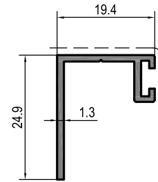
KOD: 17064 Ağırlık: 0.190 kg/mt
