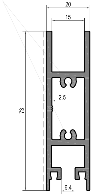
KOD: 17061 Ağırlık: 1.334 kg/mt
