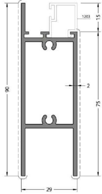
CODE / KOD 23-203-020 THEORETICAL WEIGHT kg/m TEORİK AĞIRLIK kg/m 1.275
