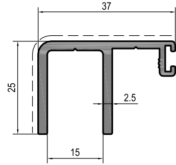
KOD: 17062 Ağırlık: 0.565 kg/mt
